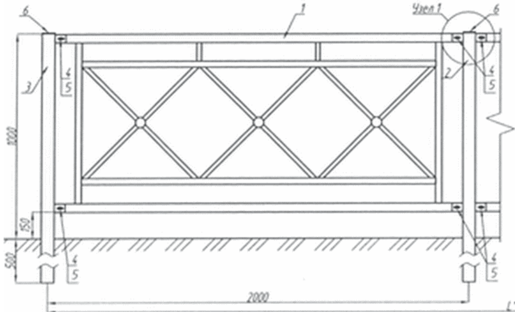
Тип 2: магистральное пешеходное ограждение безопасности
